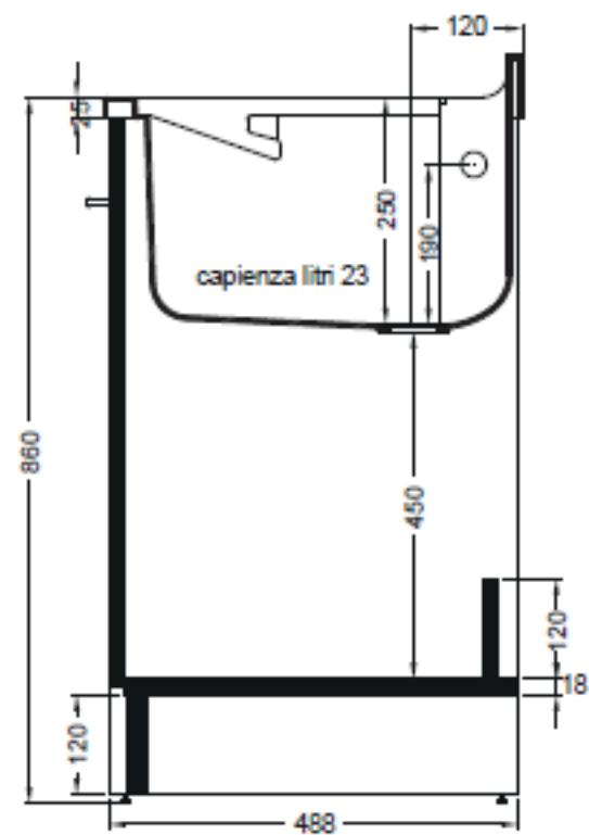
SEZIONE A-A
