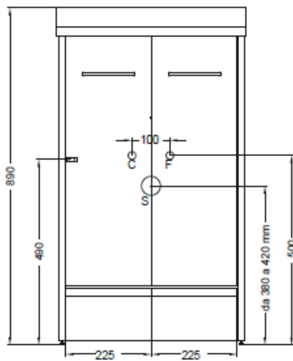
VISTA FRONTALE
