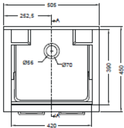
PIANTA
