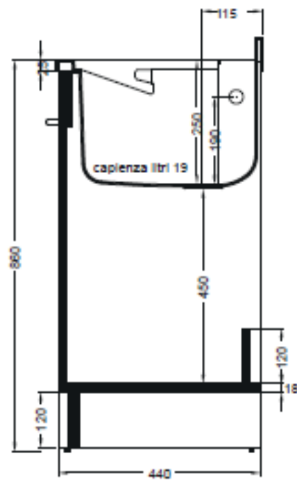
SEZIONE A-A
