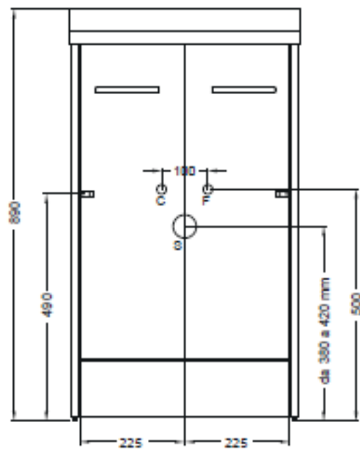
VISTA FRONTALE
