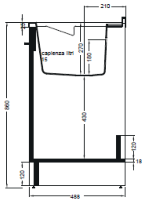
SEZIONE A-A
