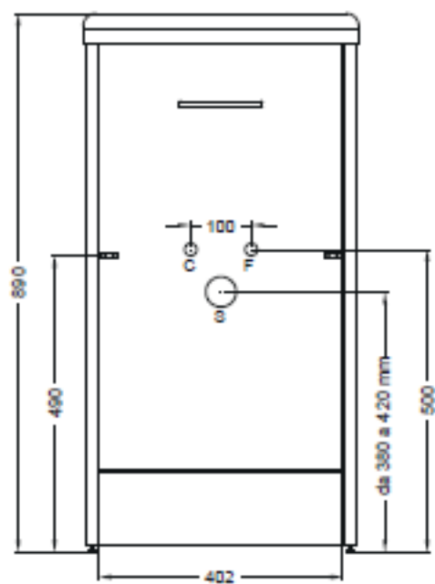
VISTA FRONTALE
